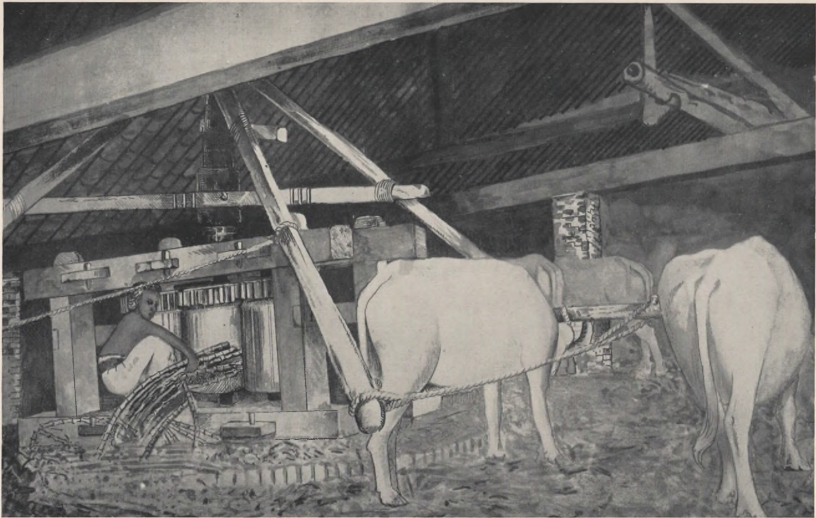
B 35. Suikermolen van Souw Siouw Keng te Paroengkoeda in het Tangerang'sche zooals deze in 1905 nog werkte. Verbleekte photo, op het terrein zelf bijgewerkt naar de aldaar nog aanwezige installatie. Vermeld in § 776. Deze molen wordt bewogen niet door karbouwen maar door zes runderen; zij draaien eene verticale ijzeren spil, waaraan een dito cylinder met een tandrad, hetwelk twee andere soortgelijke cylinders in tegengestelde richting doet draaien. Het riet wordt gestoken tusschen de twee rechtsche cylinders, komt er aan den anderen kant uit, wordt er daar ingestoken tusschen de linksche en komt aan den eersten kant uitgeperst (als ampas) te voorschijn. Het rietsap loopt in een bak en vandaar door eene leiding in een vergaarbak.
