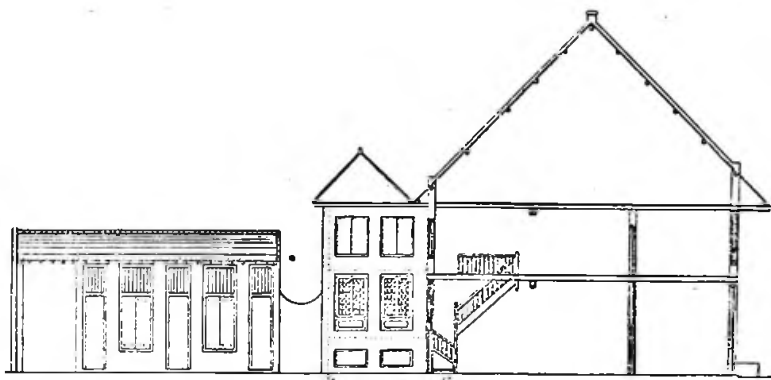
Doorsnee van het huis Spinhuisgracht No. 17 met eene van de zaal tot den achtermuur loopende plaats. Men lette op de constructie van den uitsteker.
